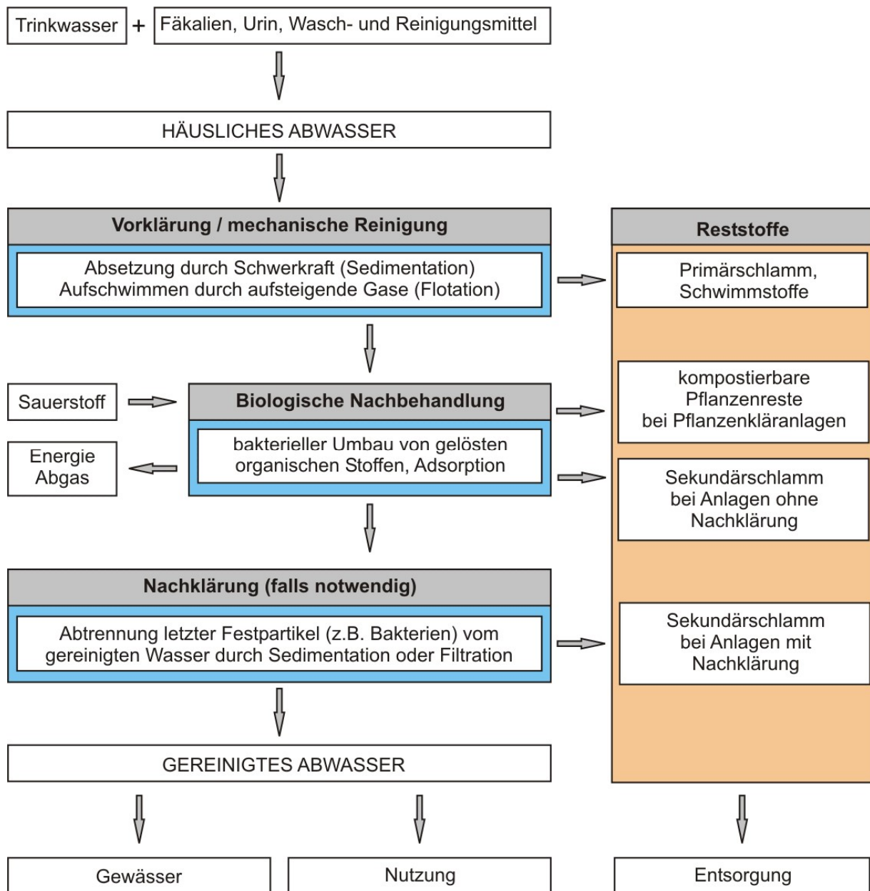
Abb.: Mechanische und biologische Reinigung in Kleinkläranlagen
