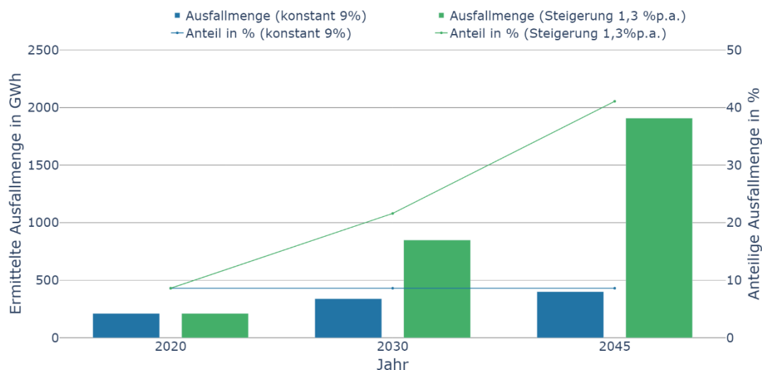
Abbildung 5: Menge und Anteil der voraussichtlich abgeregelten Windkraftanlagen in Prignitz-Oberhavel [Eigene Darstellung, Datenquelle: (REK 2021b) Regionale Energiekonzept und e.dis intern]
