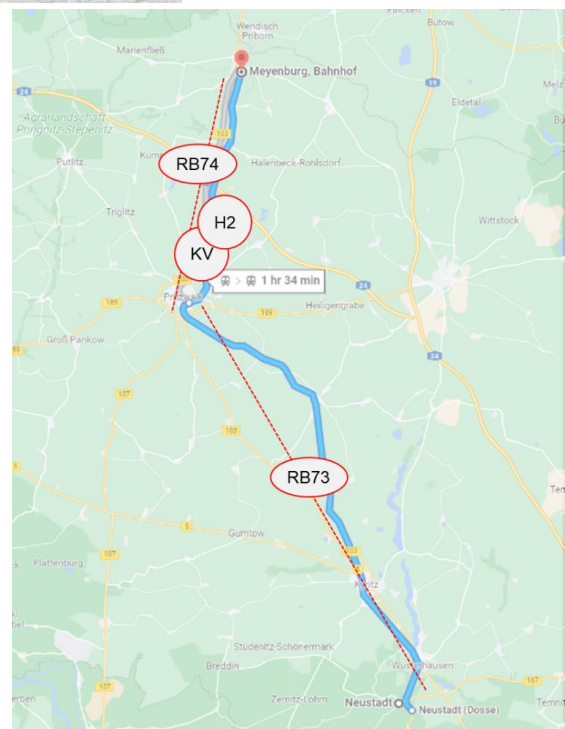
Abbildung 22: Lage Startprojekt 2. Legende: H2: Elektrolyseur; KV: Kombiverkehr-Terminal
